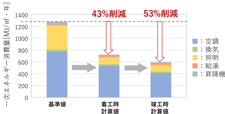
▲一次エネルギー消費量推移(オフィス)
